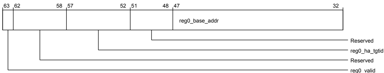
Figure 3-1058 por_cxg_ra_por_cxg_ra_sam_addr_region_reg0 (high)
