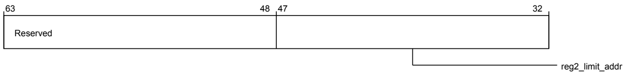
Figure 3-1078 por_cxg_ra_por_cxg_ra_sam_mem_region2_limit_reg (high)
