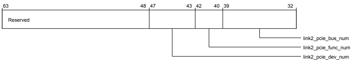
Figure 3-1196 por_cxla_por_cxla_linkid_to_pcie_bus_num (high)
