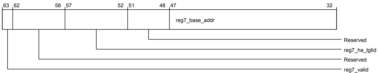
Figure 3-1072 por_cxg_ra_por_cxg_ra_sam_addr_region_reg7 (high)
