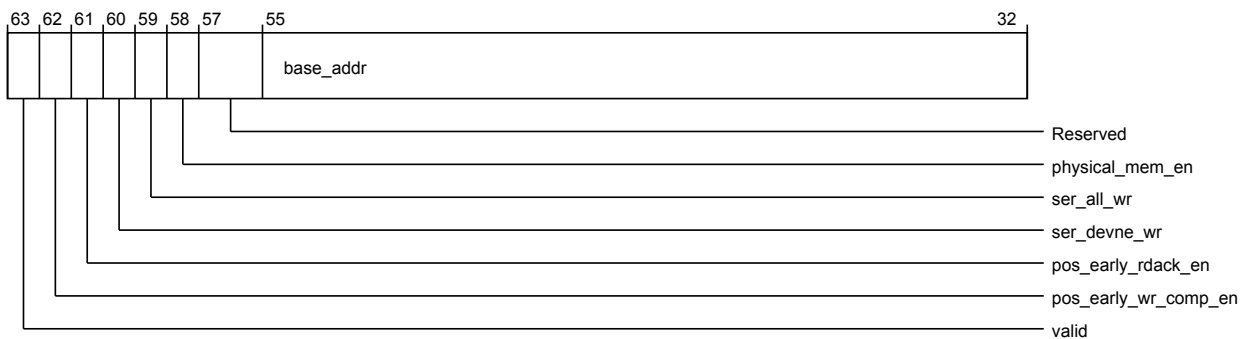
Figure 3-526 por_hni_por_hni_sam_addrregion3_cfg (high)
