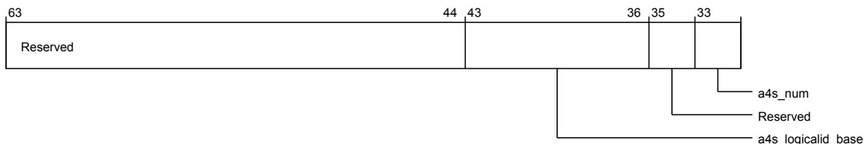
Figure 3-768 por_rni_por_rni_unit_info (high)
