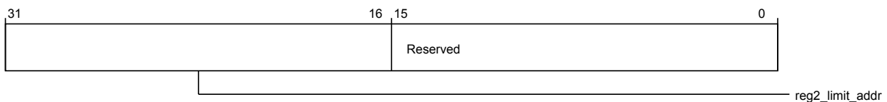
Figure 3-1079 por_cxg_ra_por_cxg_ra_sam_mem_region2_limit_reg (low)
