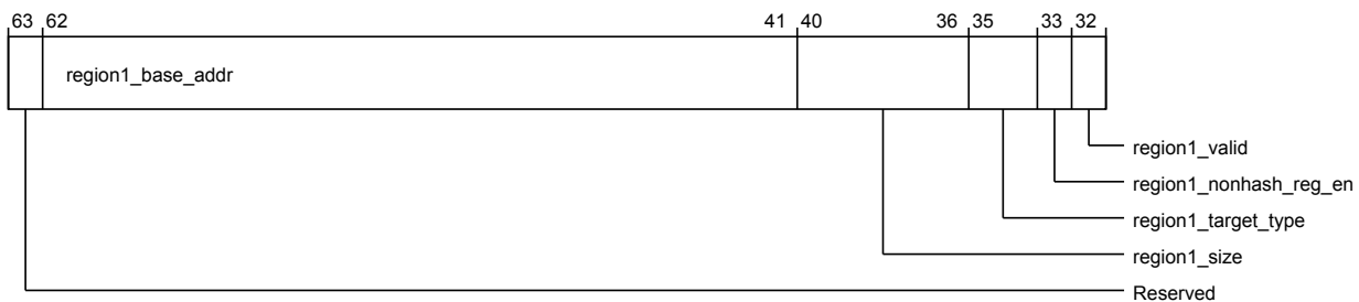
Figure 3-830 por_rnsam_sys_cache_grp_region0 (high)
