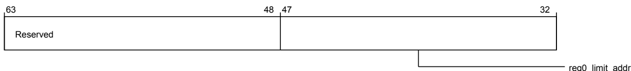
Figure 3-1074 por_cxg_ra_por_cxg_ra_sam_mem_region0_limit_reg (high)
