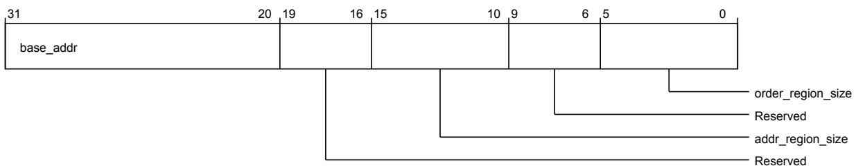
Figure 3-525 por_hni_por_hni_sam_addrregion2_cfg (low)
